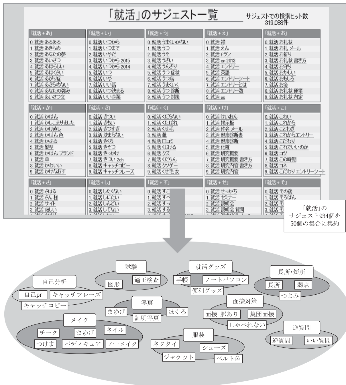
図2 検索エンジンサジェストの集約（クエリフォーカス：「就活」）
