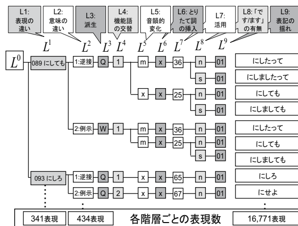
図 1: 形態素に基づく階層構造
