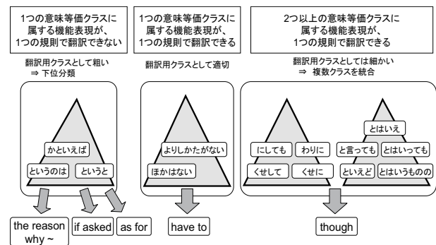
図 4: 意味等価クラスの粒度の再編
