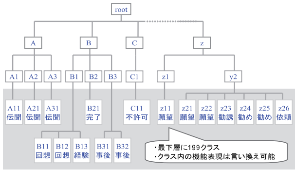
図 2: 意味等価クラス
